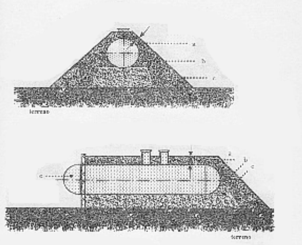
TAVOLA 1 C: SERBATOIO RICOPERTO CON CALOTA ESTERNA AL MANTO DI RICOPRIMENTO
