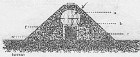
TAVOLA 1 E: SERBATOI RICOPERTI CON CUNCCIO DI ACCESSO A PARTE DELLA CALOTA
