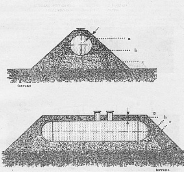
TAVOLA 1 B: SERBATOIO TOTALMENTE RICOPERTO
