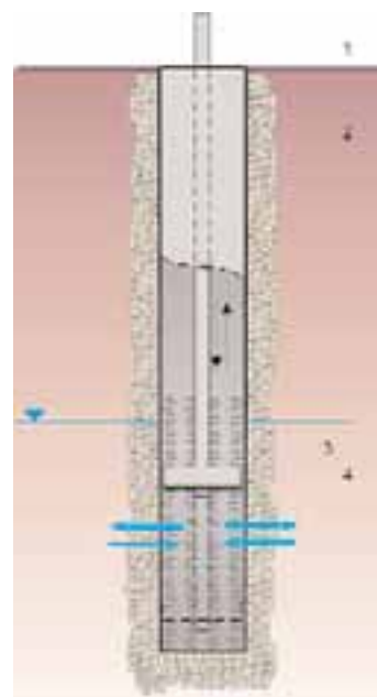
Figura 3.25 - Schema di sviluppo mediante pistonaggio: 1) asta pesante; 2) rivestimento; 3) filtri; 4) pistone
