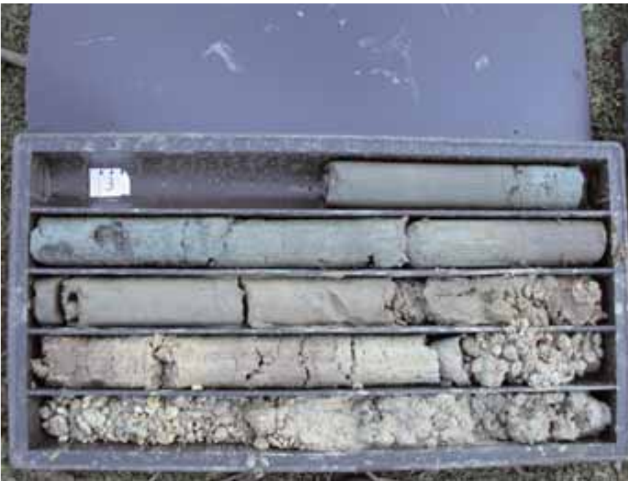
Figura 2.22 - Cassetta catalogatrice con carota di terreno. Può essere di legno o materiale plastico e serve a riporre la carota per tutto il tempo necessario al geologo di campo per effettuare il prelievo di campioni di terreno o gas interstiziali, l'analisi delle proprietà organolettiche, le valutazioni sul tipo di granulometria e grado di umidità e, da ultimo, le foto. Le cassette devono recare, oltre al codice del sondaggio di provenienza, l'indicazione dell'intervallo di profondità carotato (ad es. da 0 a 4 m) e, possibilmente, delle profondità parziali di ciascuno spezzone di carota contenuto. Nel caso non venga espressamente richiesto di conservare la carota, questa può essere impiegata per riempire il foro di sondaggio o smaltita secondo quanto previsto dalle norme
