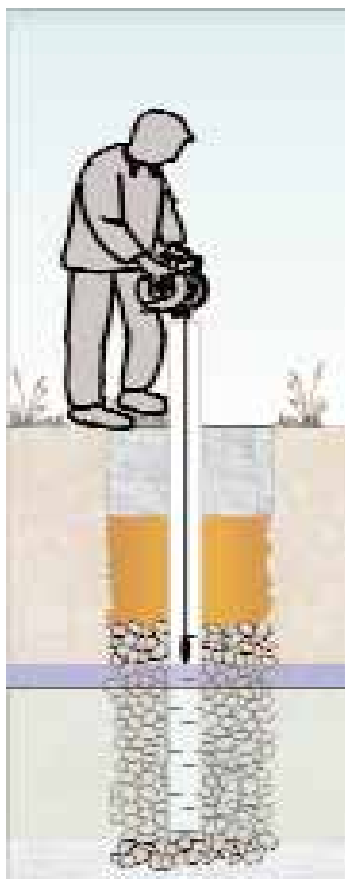
Figura 3.28 - Schema di utilizzo del freatimetro
