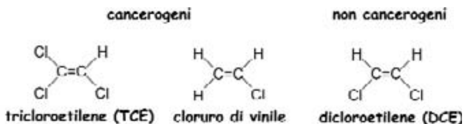
Figura 8.25 - Alcuni esempi di struttura di alifatici clorurati. Questi composti sono costituiti da idrocarburi in cui uno o più atomi di H sono sostituiti da atomi di Cl
