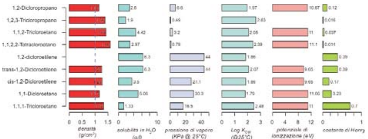
Figura 8.27 - Caratteristiche chimico-fisiche degli idrocarburi alifatici clorurati non cancerogeni. Si osserva che generalmente la densità della sostanza è direttamente proporzionale alla presenza degli atomi di cloro
