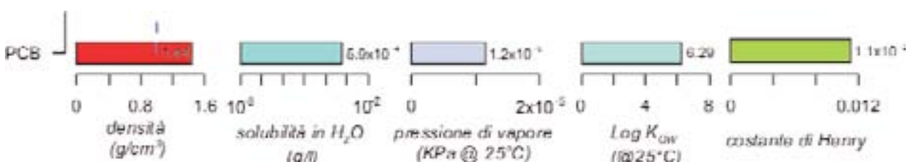
Figura 8.43 - Caratteristiche chimico-fisiche dei PCB. I valori riportati sono indicativi dei congeneri più diffusi
