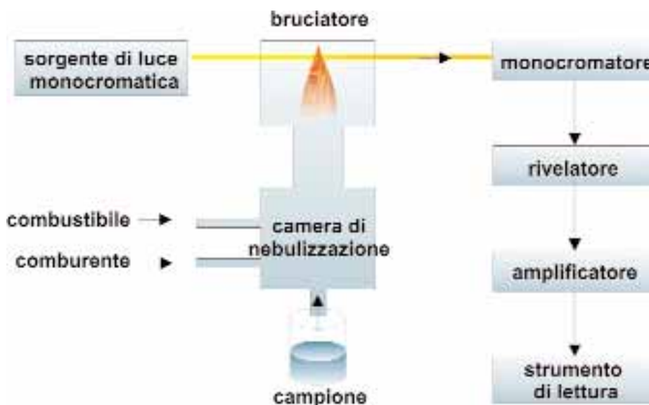
Figura 8.6 - Spettrometria di assorbimento atomico con atomizzazione a fiamma (FAAS) o con fornetto di grafite (GFAAS). Nella spettrometria FAAS la soluzione da analizzare viene nebulizzata ed avviata verso una fiamma (bruciatore) che atomizza i singoli elementi presenti nella soluzione stessa. Nel caso della GFAAS il bruciatore è costituito da un cilindro di grafite, riscaldato elettricamente, a temperature nell'ordine dei 2800°C. Per ogni elemento da analizzare un raggio luminoso monocromatico dotato di una energia iniziale attraversa il bruciatore e intercettando gli atomi viene in parte assorbito. Il rapporto fra energia posseduta dal raggio luminoso in entrata e in uscita dal bruciatore è proporzionale alla concentrazione dell'elemento da determinare. La determinazione della concentrazione è quindi ottenuta attraverso la costruzione di una retta di calibrazione con opportune soluzioni standard
