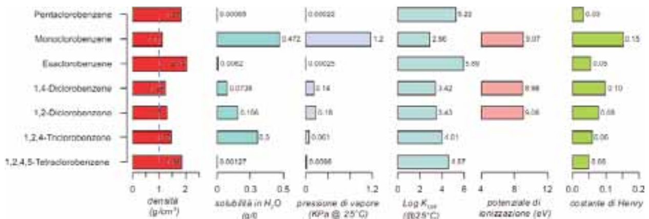
Figura 8.33 - Caratteristiche chimico-fisiche dei clorobenzeni. Sono caratterizzati da densità piuttosto elevate e alcune specie anche da elevata solubilità e volatilità. Si osserva che generalmente la densità della sostanza è direttamente proporzionale alla presenza degli atomi di Cl
