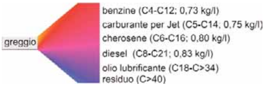
Figura 8.48 - Attraverso la raffinazione del greggio che comprende processi quali la distillazione, l'alchilazione (processo atto ad aumentare il numero di ottani), il reforming, (sintesi per ottenere idrocarburi più pesanti a partire da molecole più leggere) o cracking (l'inverso del reforming) si ottiene la vasta gamma di specie necessarie per realizzare i prodotti finali di idrocarburi, che si distinguono per densità, viscosità, potere calorifico, punti di ebollizione, numero di atomi di C specifici. La composizione di questi prodotti comprende anche alcuni additivi (es. ammine, fenoli, metalli, alcool, ecc.) aventi funzioni specifiche (inibitori della corrosione, antiossidanti, migliorativi delle performance, ecc.)
