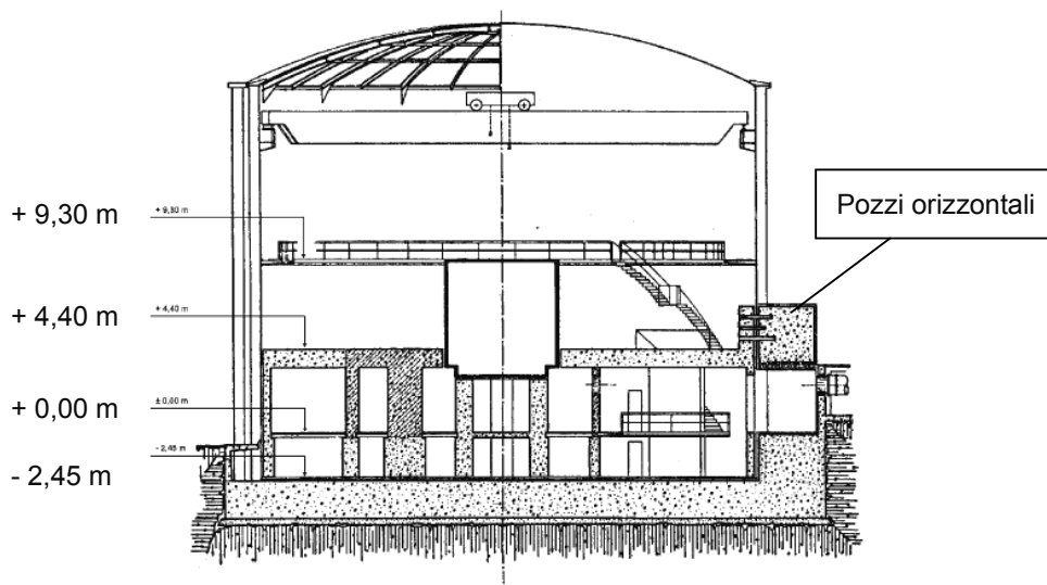
Figura 3 - Edificio di contenimento del reattore
