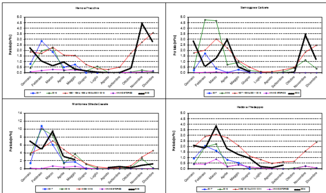
fig.16: Andamento delle portate medie mensili di alcuni affluenti del Reno e di alcuni Fiumi Romagnoli, messo a confronto con l'anno precedente 2016 e con valori di lungo periodo, quali la media ed il minimo storico
