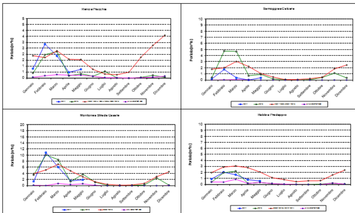
Fig.11: Andamento delle portate medie mensili di alcuni affluenti del Reno e di alcuni Fiumi Romagnoli, messo a confronto con l'anno precedente 2016 e con valori di lungo periodo, quali la media ed il minimo storico
