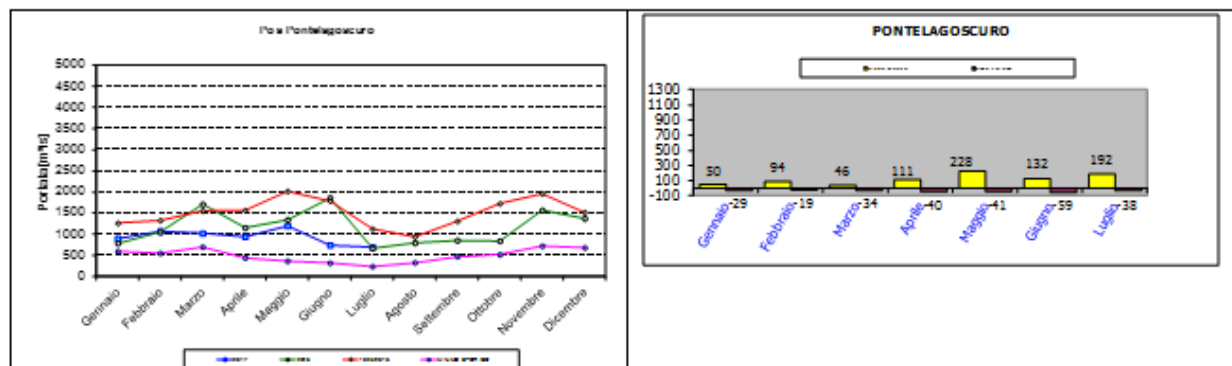
Fig.17: Nell'immagine di sinistra viene riportato l'andamento delle portate medie mensili del Po a Pontelagoscuro messo a confronto con l'anno precedente 2016 e con valori di lungo periodo, quali la media ed il minimo storico; nell'immagine di destra viene fornito l'andamento mensile dello scarto percentuale di tali valori di portata dalle medie di lungo periodo e dai minimi storici mensili
