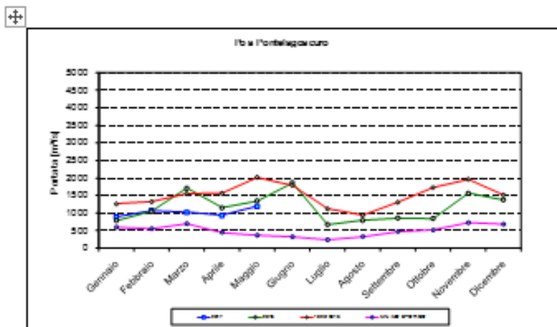
Fig.12: Andamento delle portate medie mensili del Po a Pontelagoscuro messo a confronto con l'anno precedente 2016 e con valori di lungo periodo, quali la media ed il minimo storico.
