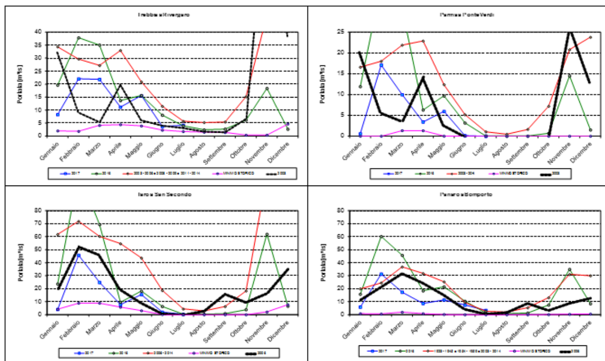
fig.10: Andamento delle portate medie mensili di alcuni affluenti emiliani del Po, posto a confronto con l'anno precedente 2016 e con valori di lungo periodo, quali la media ed il minimo storico
