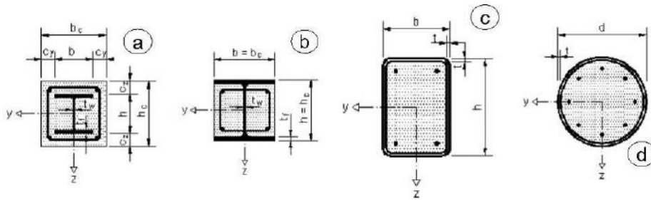
Fig. 4.3.6 - Tipi di sezioni per colonne composte, trattate nel presente paragrafo .
