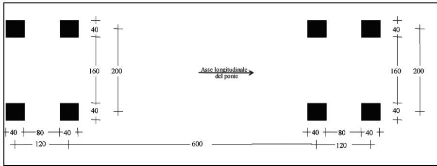
Fig. 5.1.5 - Modello di carico di fatica. 3
