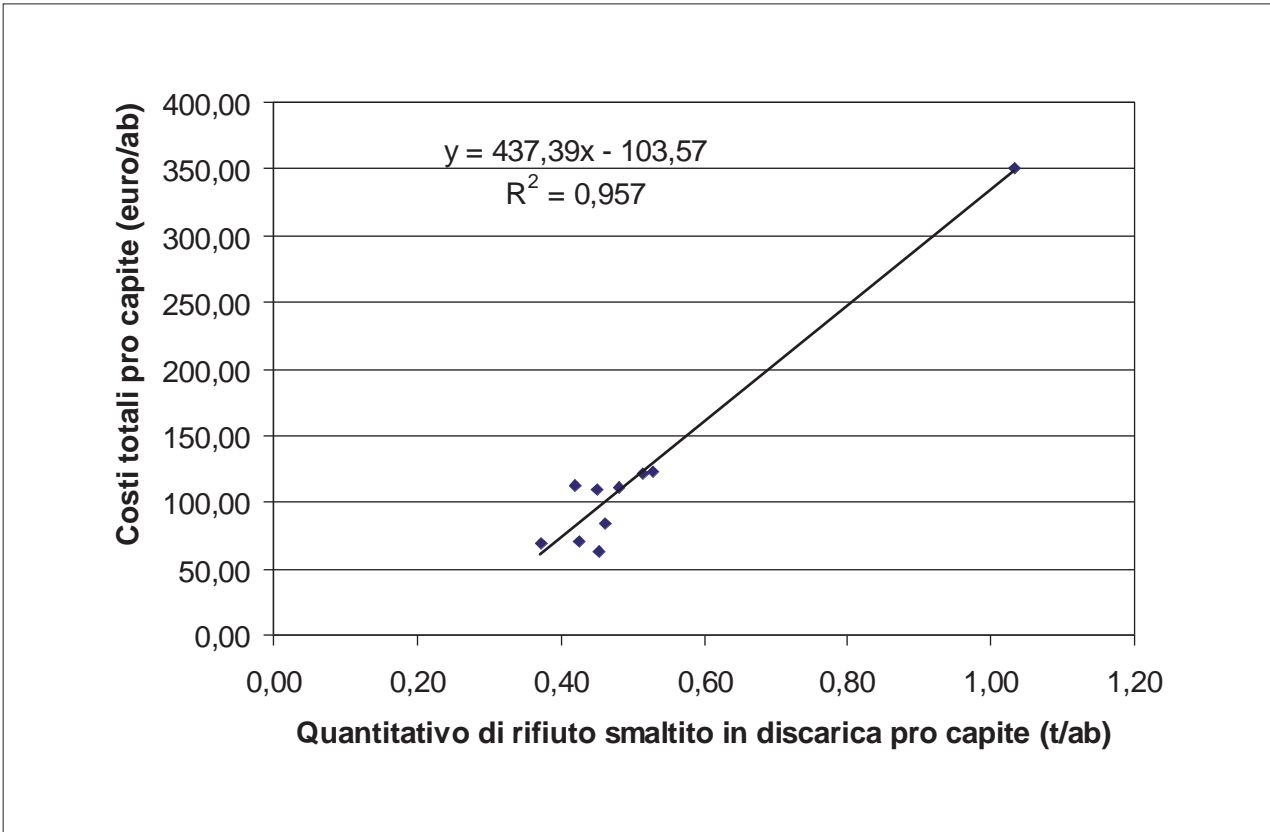
Figura 4.18 - Andamento dei costi totali pro capite (€/ab) di gestione del servizio di igiene pubblica in funzione del quantitativo pro capite di rifiuti smaltito in discarica (t/ab) con valori di “% disc” > 80%, anno 2005
