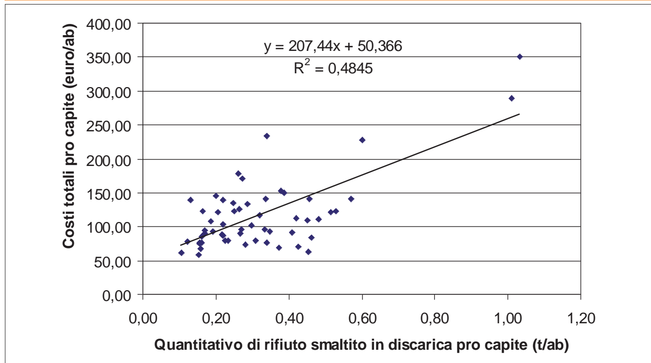
Figura 4.14 - Andamento dei costi totali pro capite (€/ab) di gestione del servizio di igiene pubblica in funzione del quantitativo pro capite di rifiuti smaltito in discarica (t/ab) con valori di “% disc” > 30%, anno 2005
