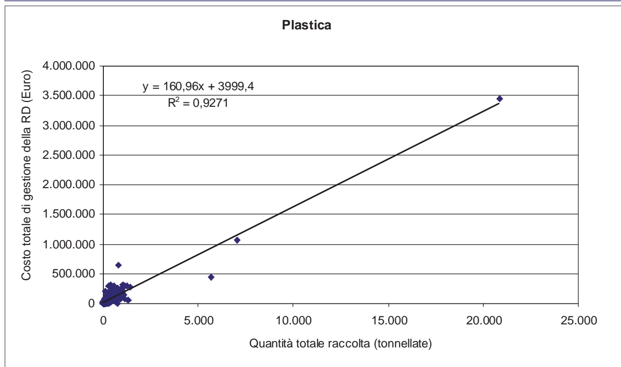
Figura 5.21 - Andamento dei costi totali di raccolta della plastica in funzione delle quantità totali raccolte
