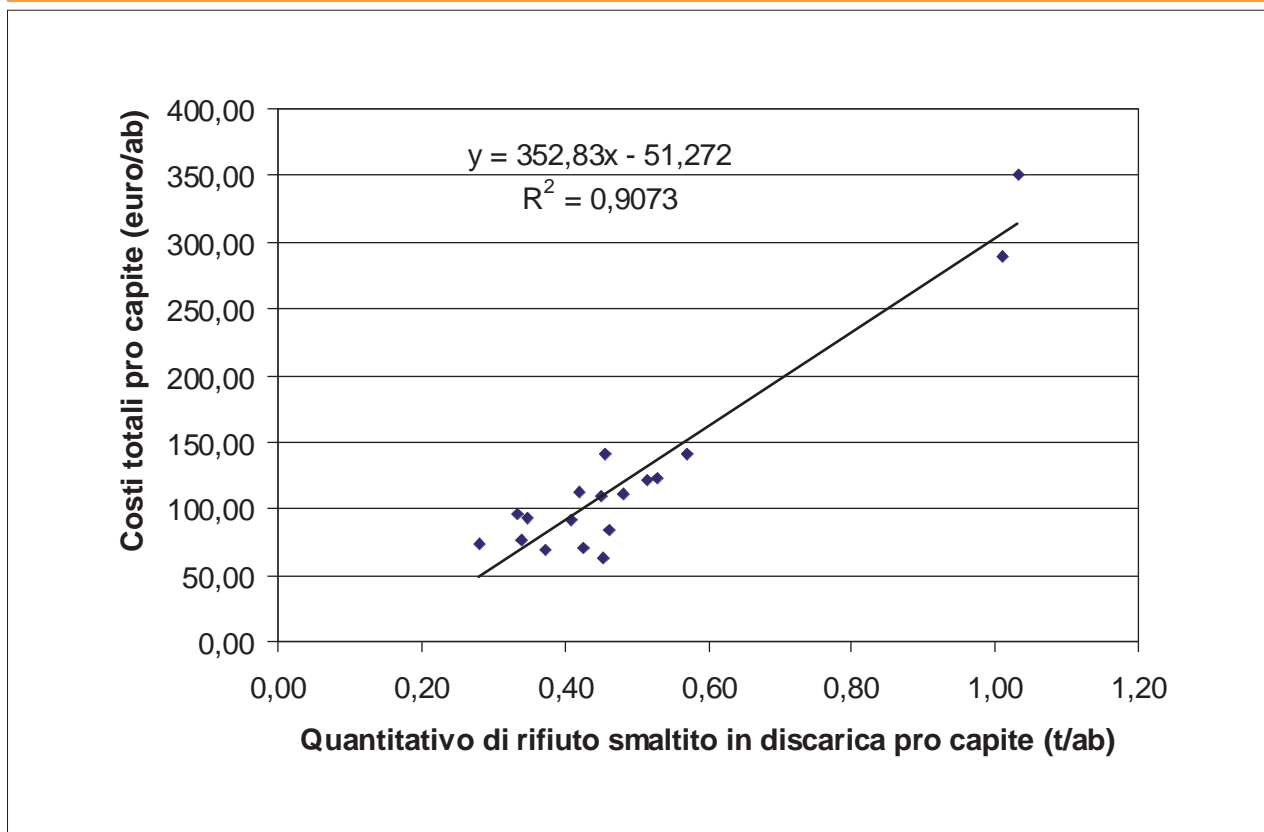
Figura 4.17 - Andamento dei costi totali pro capite (€/ab) di gestione del servizio di igiene pubblica in funzione del quantitativo pro capite di rifiuti smaltito in discarica (t/ab) con valori di “% disc” > 60% , anno 2005
