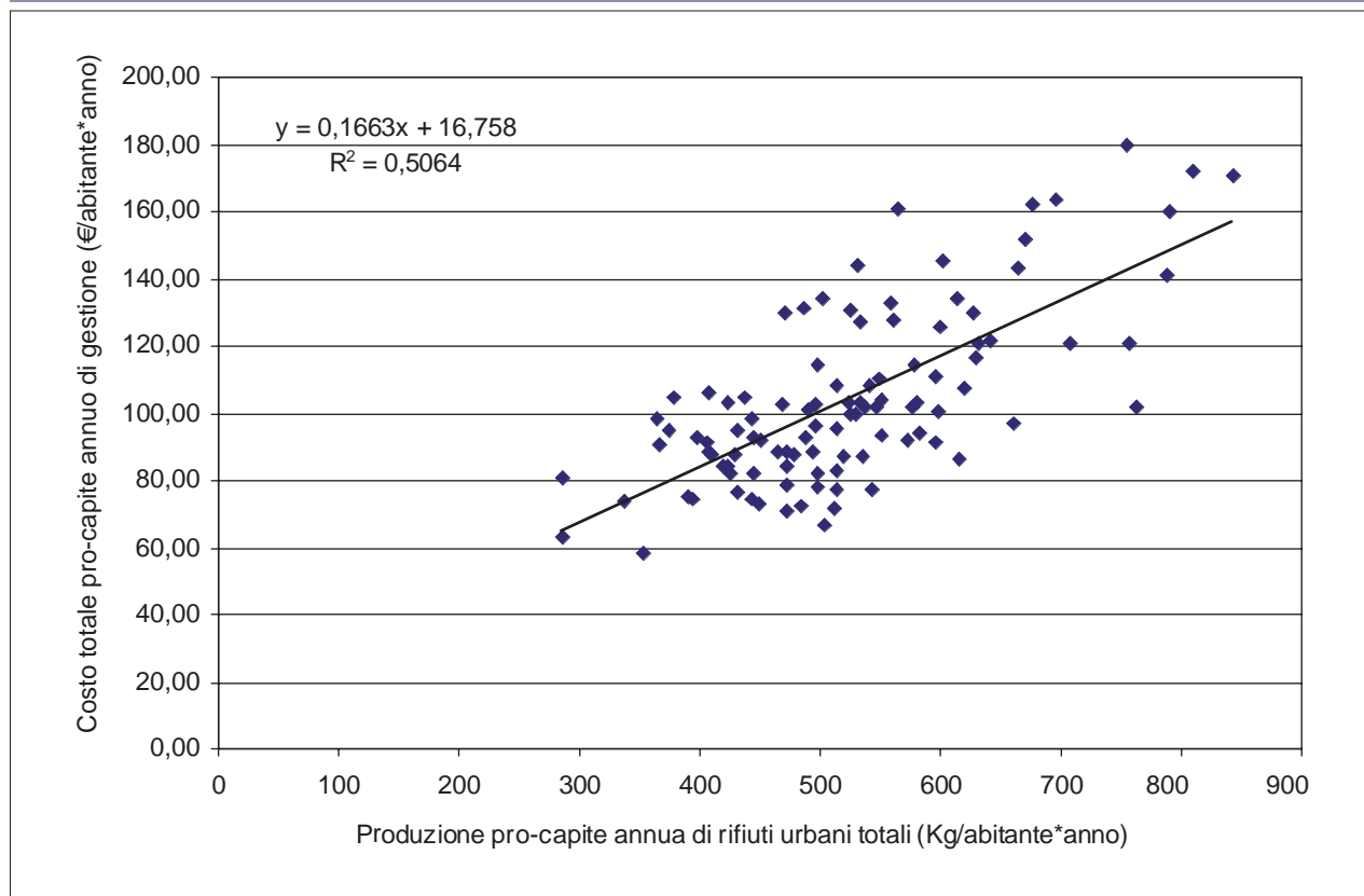
Figura 5.9 – Andamento del costo totale pro capite annuo (euro/abitante per anno) con la quantità pro-capite di rifiuti totali prodotti (kg/abitante per anno)
